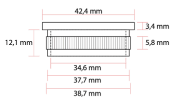
Vista laterale
